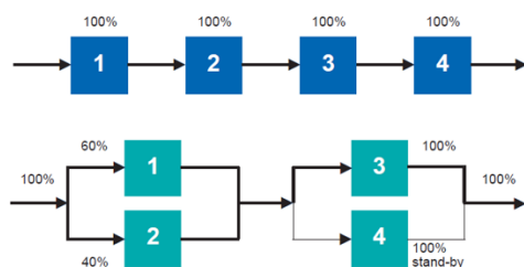
4. sz. ábra: Soros és párhuzamos gyártási technológia
